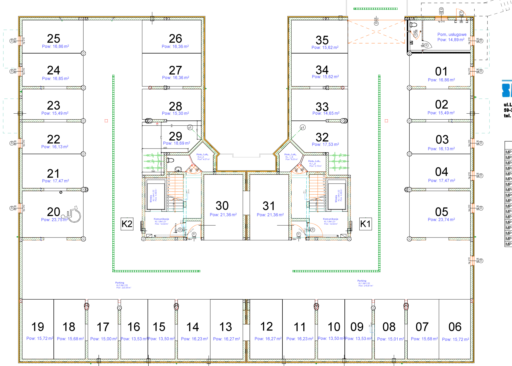
RZUT GARAŻU WIELOSTANOWISKOWEGO
