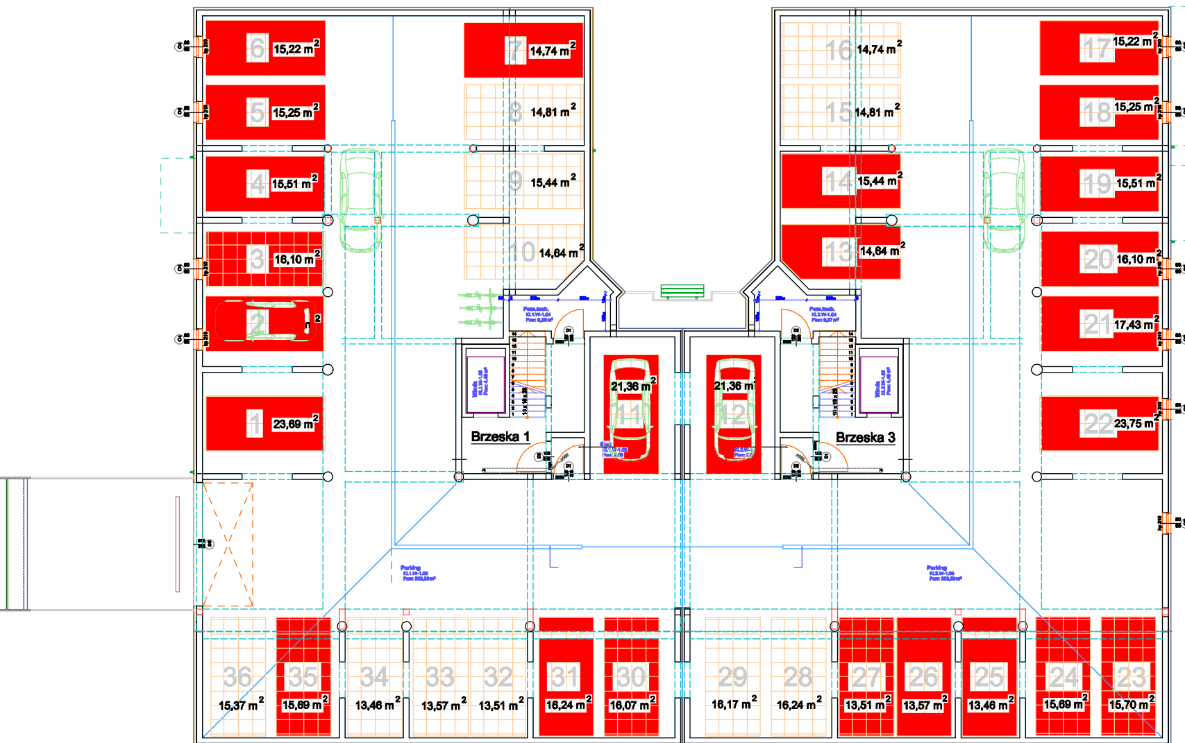
Rzut garażu wielostanowiskowego
