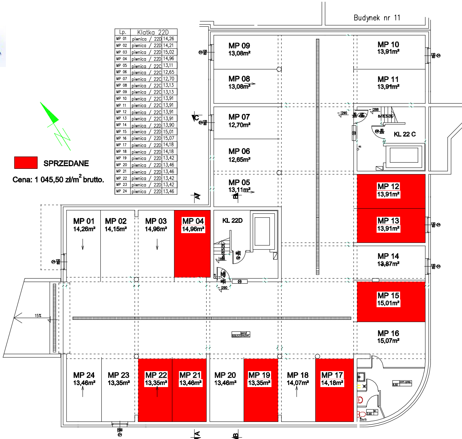
BUDYNEK MIESZKALNY WIELORODZINNY KRZEMIENIECKA 22C,D RZUT GARAŻU
